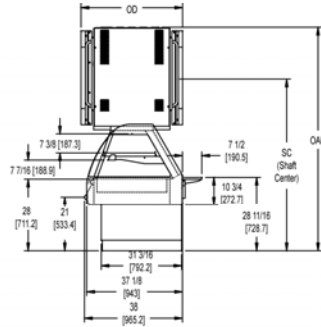
END VIEW (VGGTSWG-3, 4 & 5)
