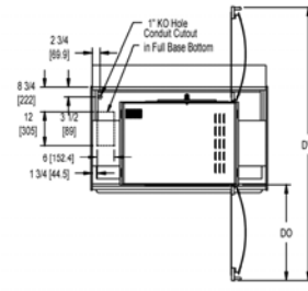
TOP VIEW (VGGTSWG-3, 4 & 5)
